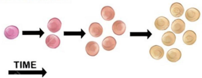
LINEAR EVOLUTION
